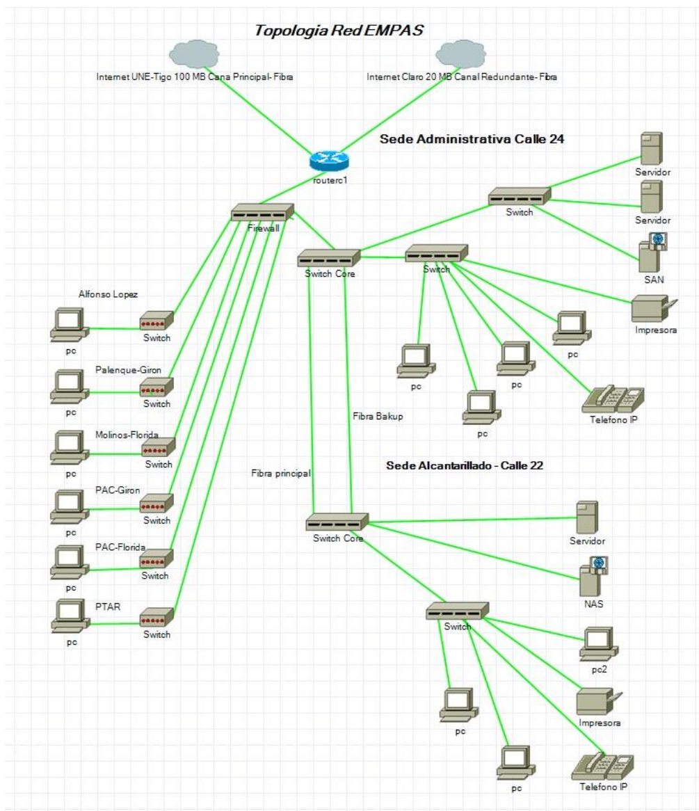
Gráfica 3. Diagrama de red de EMPAS S.A.
