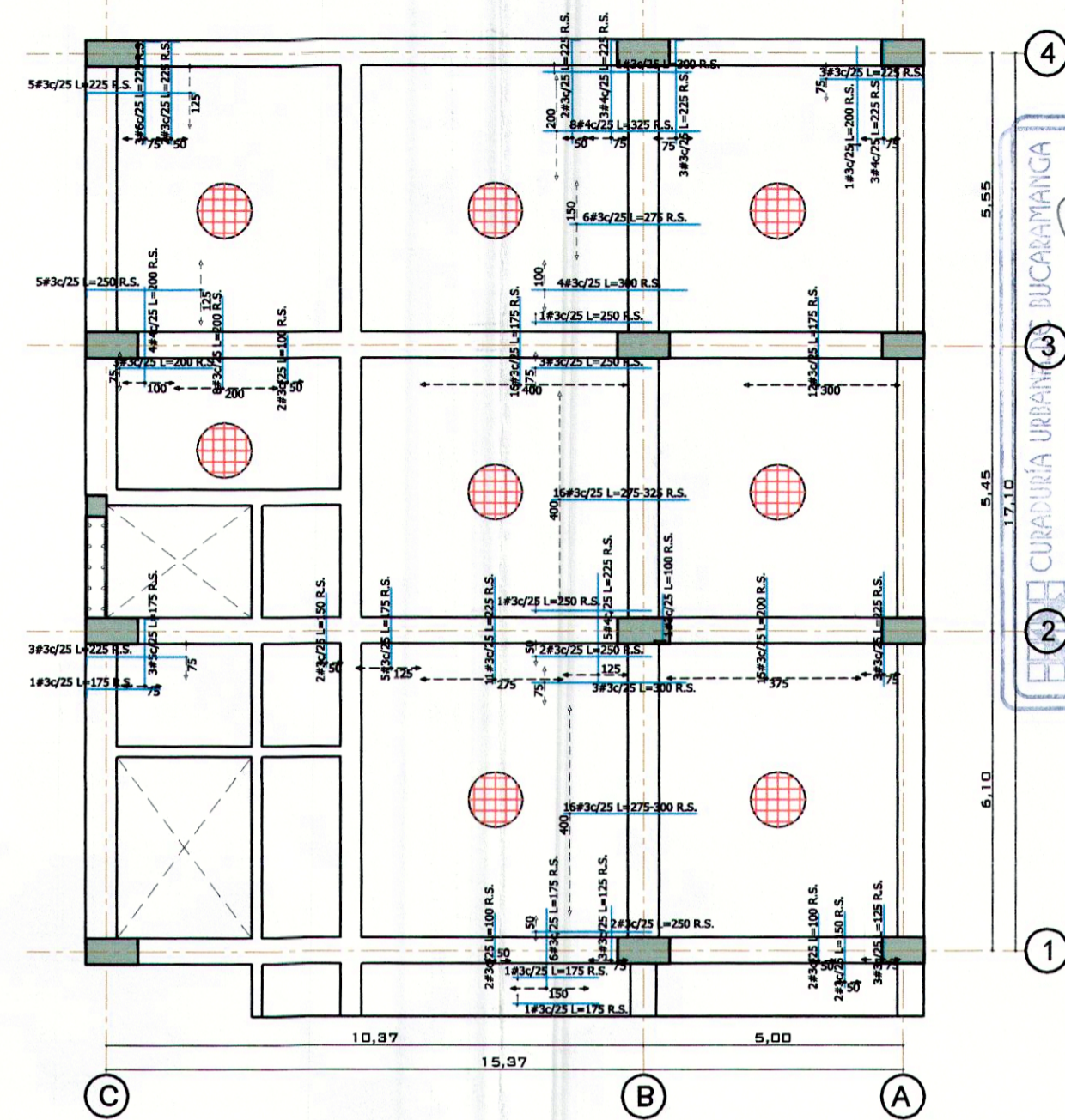
PLANTA PISO 6 A B REFUERZO SUPERIOR Y ADICIONAL ESC: 1:125
