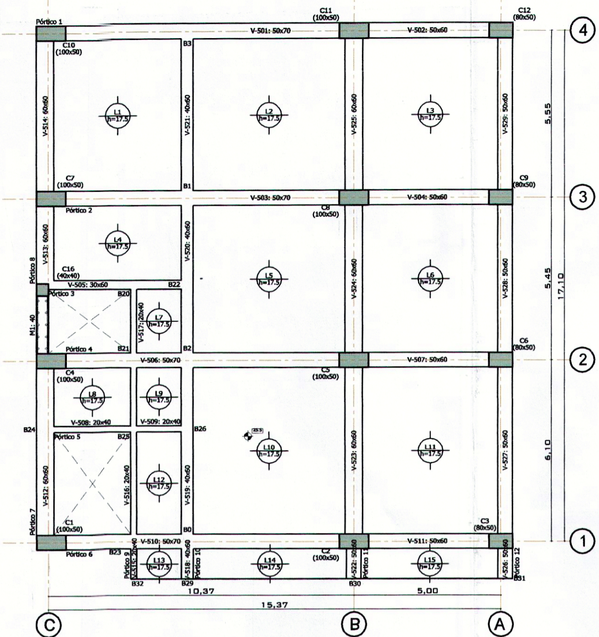
PLANTA PISO 6 A B ESC: 1:125
