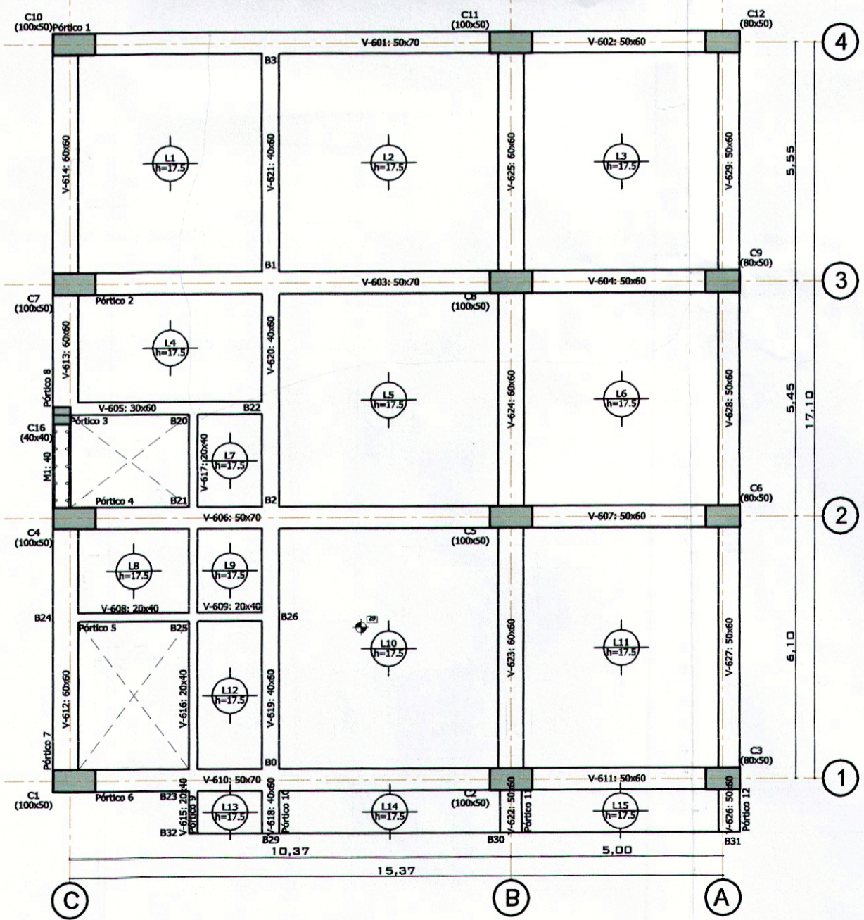
PLANTA PISO 9 ESC: 1:125
