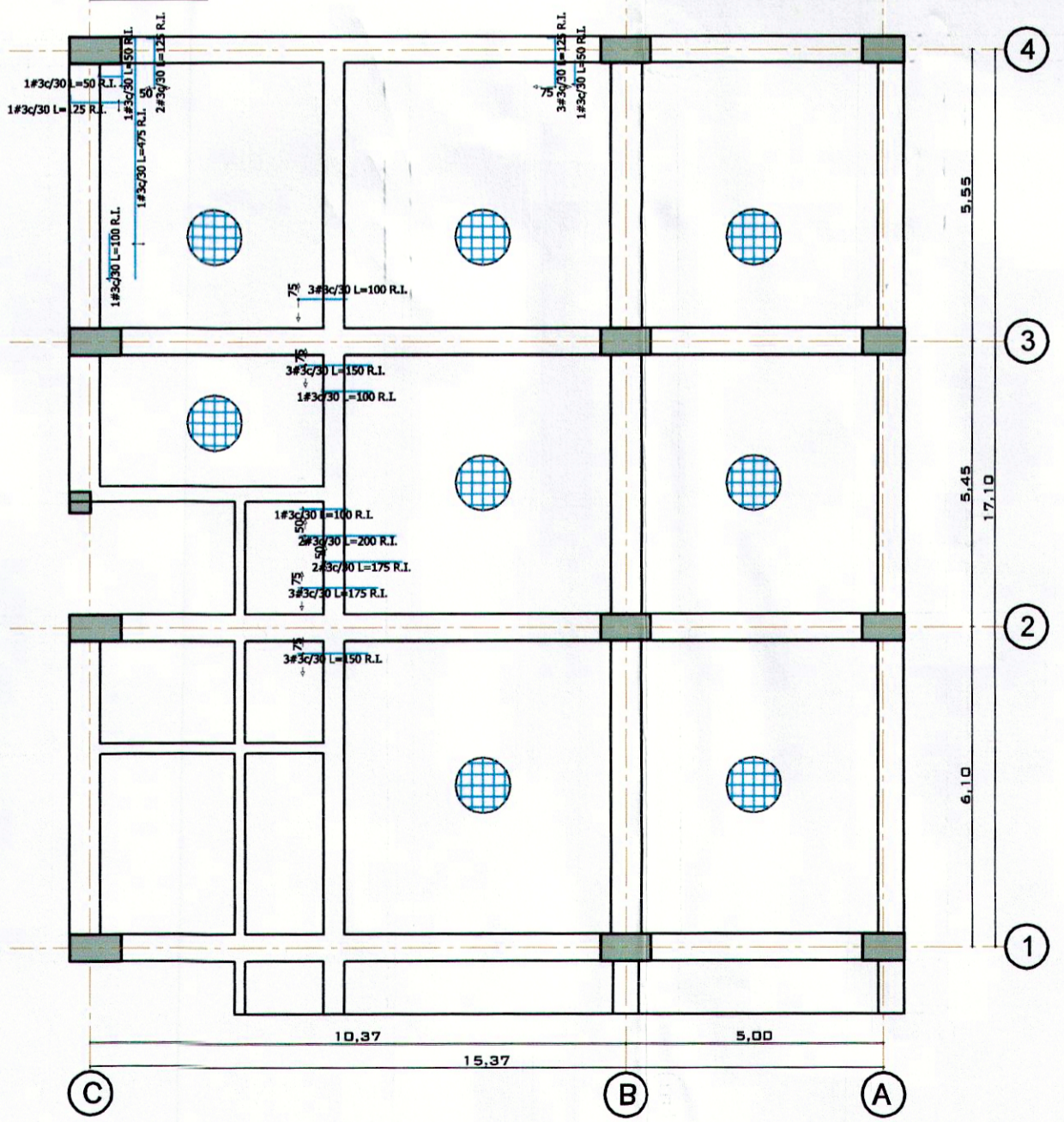
PLANTA PISO 9 REFUERZO INFERIOR Y ADICIONAL ESC: 1:125
