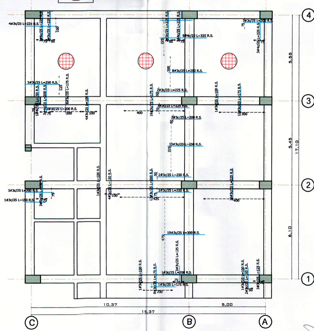
PLANTA PISO 9 REFUERZO SUPERIOR Y ADICIONAL ESC: 1:125
