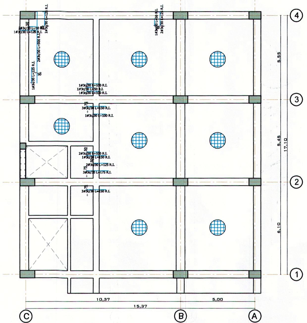
PLANTA PISO 6 A B REFUERZO INFERIOR Y ADICIONAL ESC: 1:125
