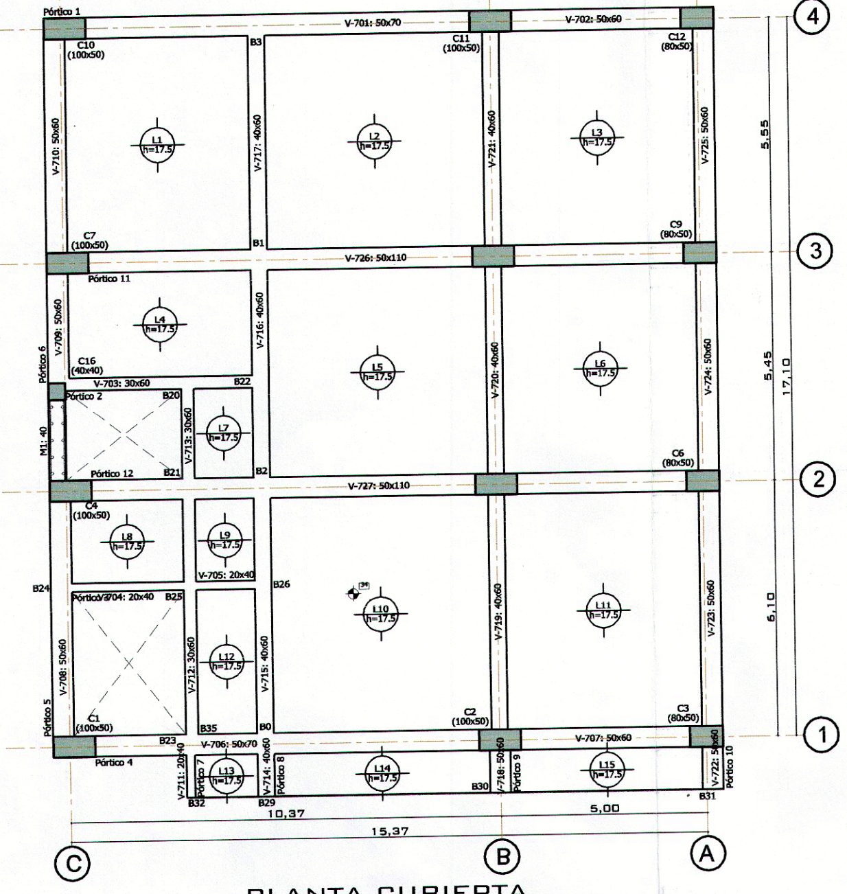
PLANTA CUBIERTA ESC: 1:125
