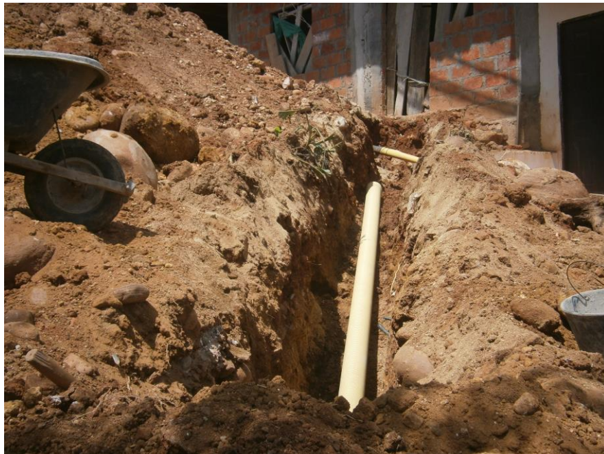
FOTO 3 – INSTALACION DE TUBERÍA SANITARIA – 15 DE SEPTIEMBRE DE 2014
